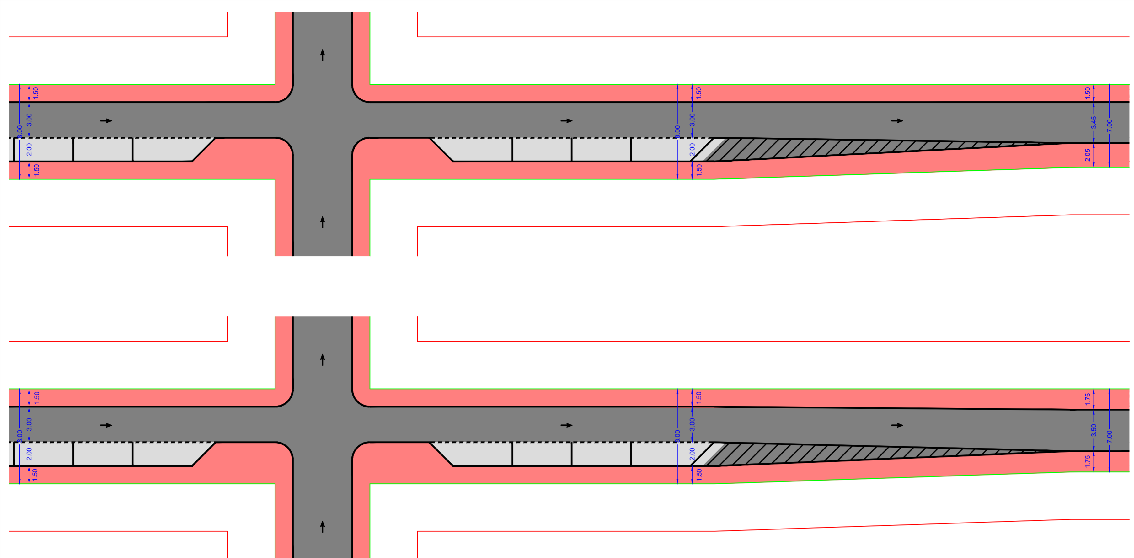
ΛΕΠΤΟΜΕΡΕΙΕΣ ΣΥΝΑΡΜΟΓΗΣ - ΚΛΙΜΑΚΑ 1:200
